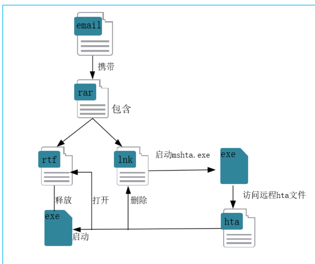
图 8. “钓鱼”邮件攻击过程示意图
