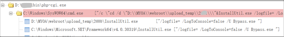
图 9. 台 APT 组织利用国内某办公自动化系统（OA）漏洞进行攻击
