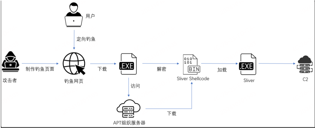
图 1. APT-C-01 组织攻击技战术示意图
